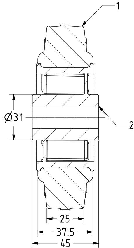
SECTION A-A
