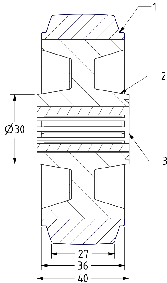
SECTION A-A
