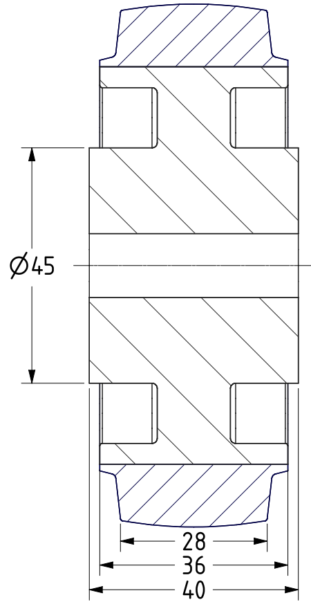
SECTION A-A
