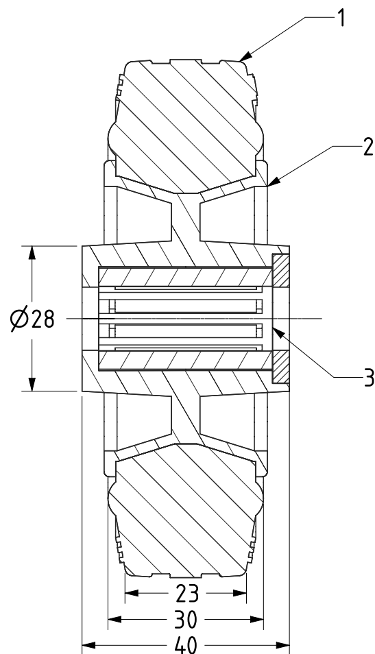
SECTION A-A
