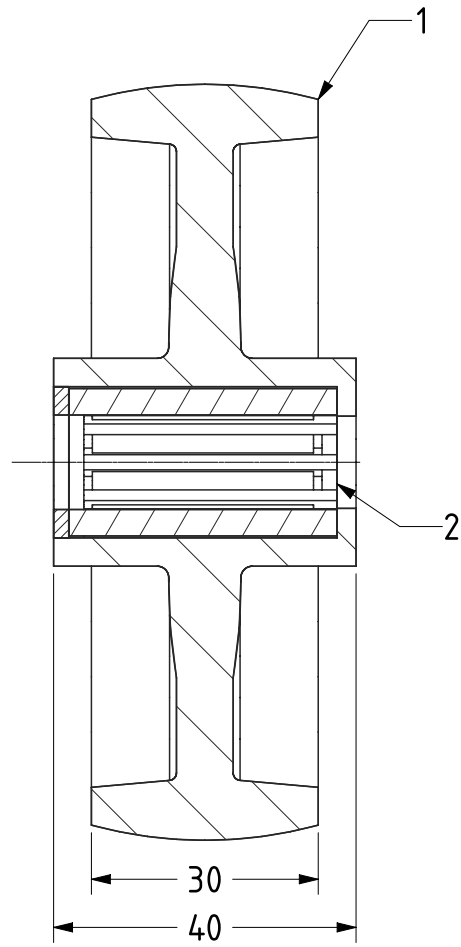
SECTION A-A
