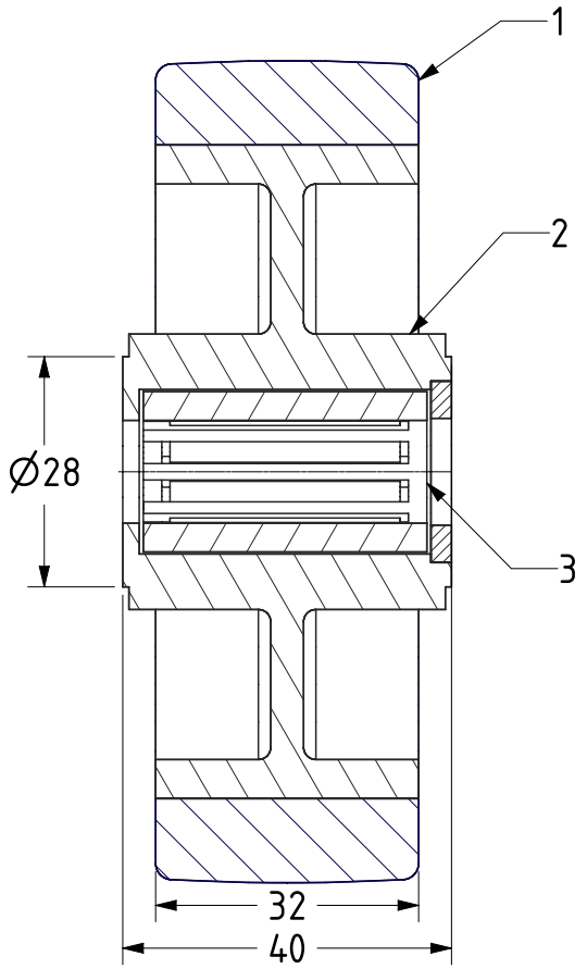
SECTION A-A
