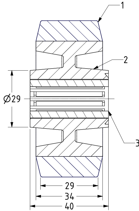
SECTION A-A
