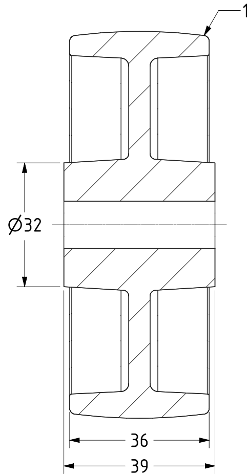
SECTION A-A
