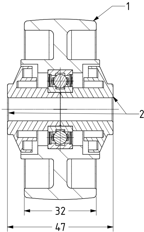
SECTION A-A
