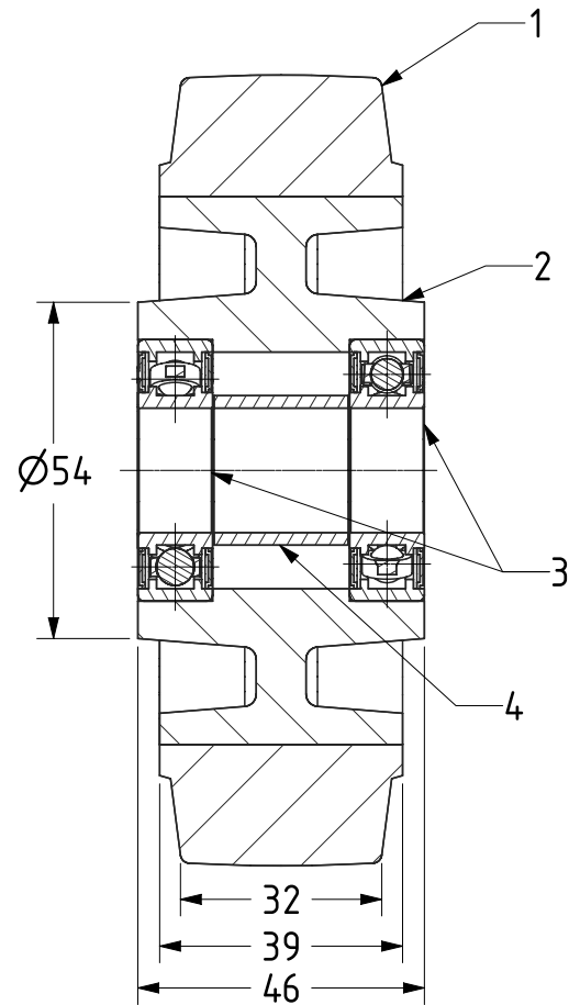
SECTION A-A
