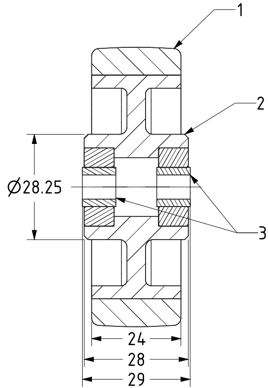
SECTION A-A
