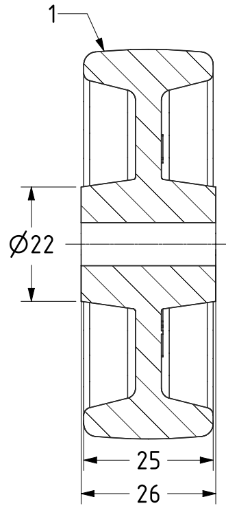
SECTION A-A
