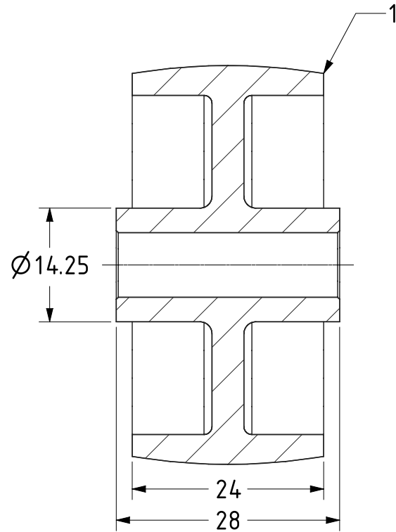
SECTION A-A
