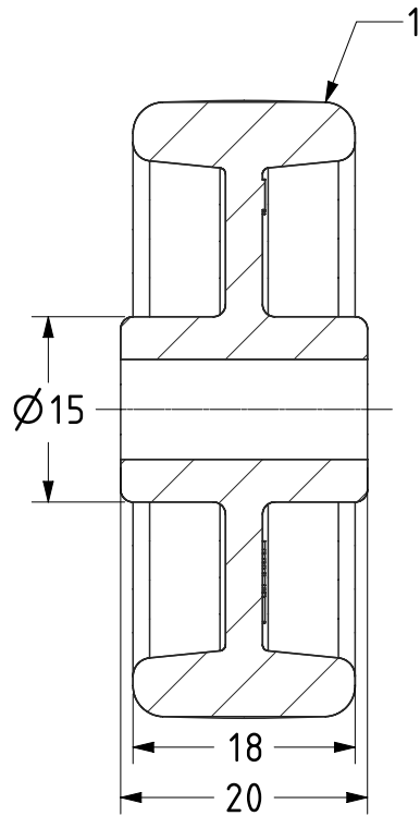
SECTION A-A
