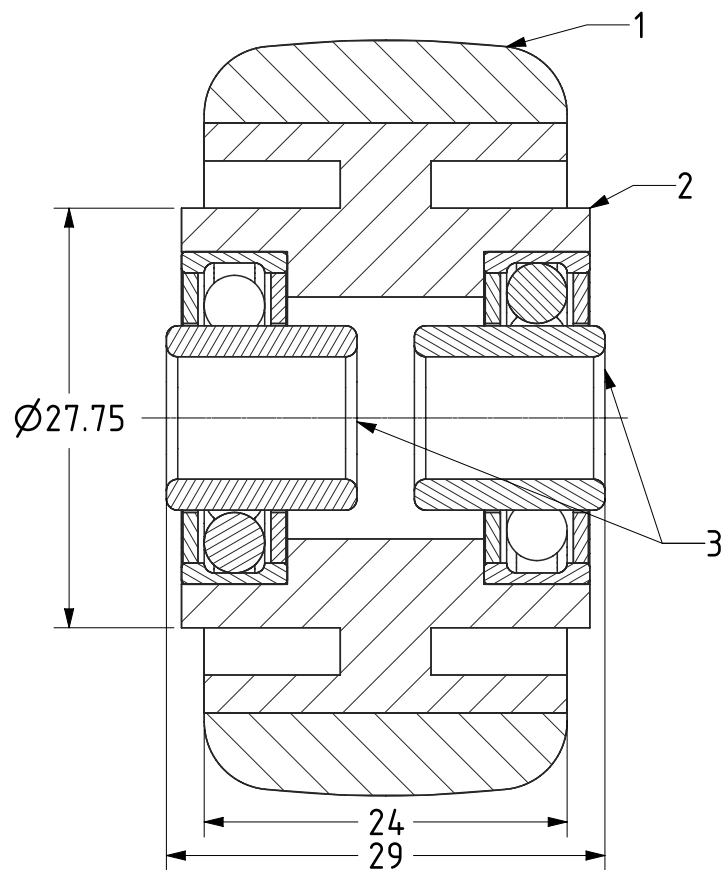
SECTION A-A
