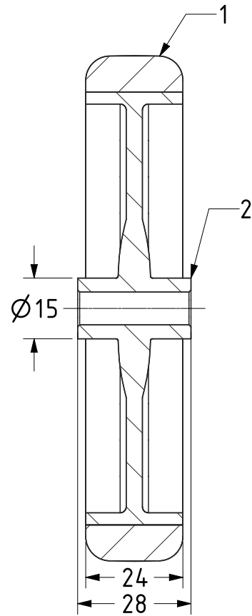
SECTION A-A
