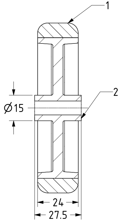
SECTION A-A
