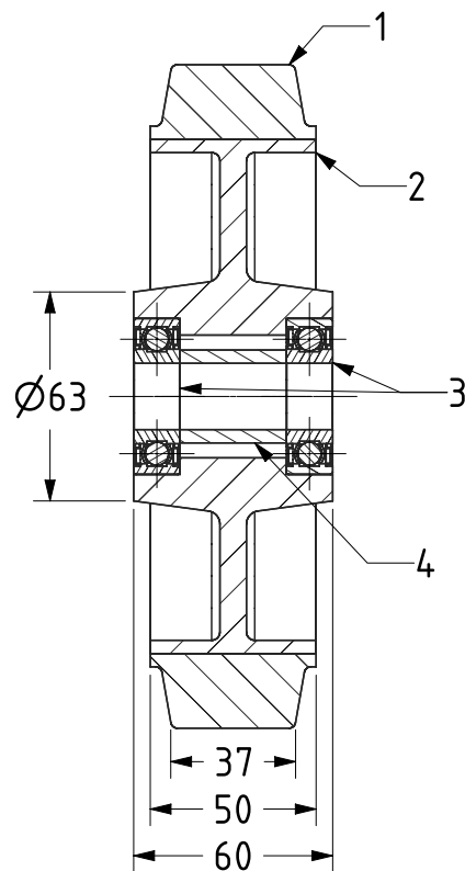
SECTION A-A
