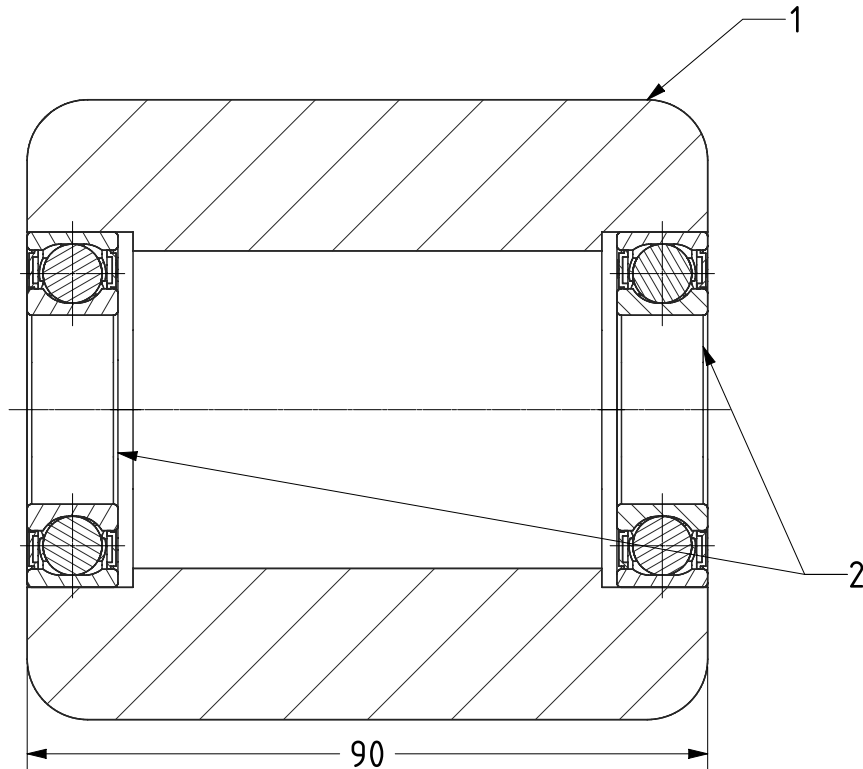
SECTION A-A
