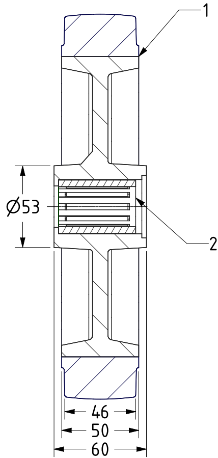
SECTION A-A
