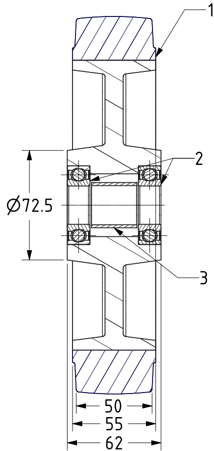
SECTION A-A
