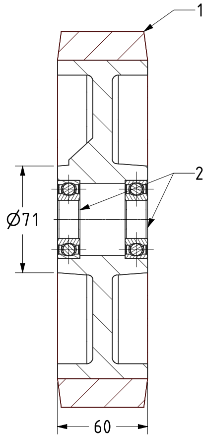
SECTION A-A
