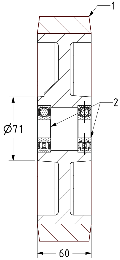
SECTION A-A
