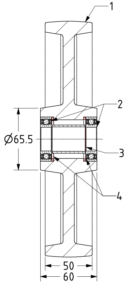
SECTION A-A
