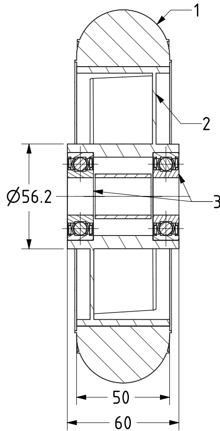
SECTION A-A
