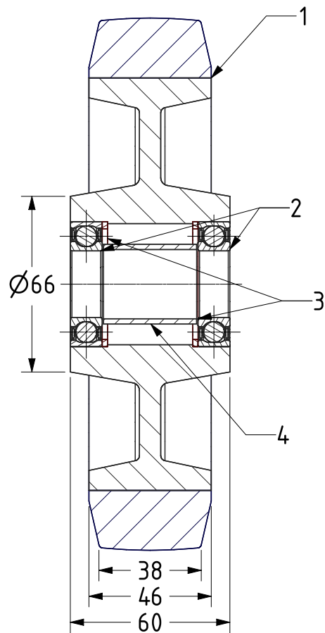
SECTION A-A
