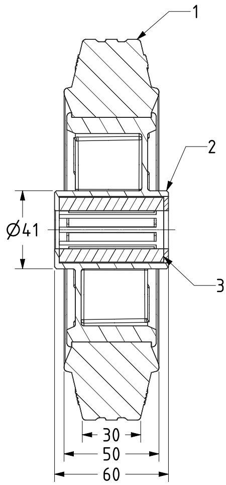
SECTION A-A
