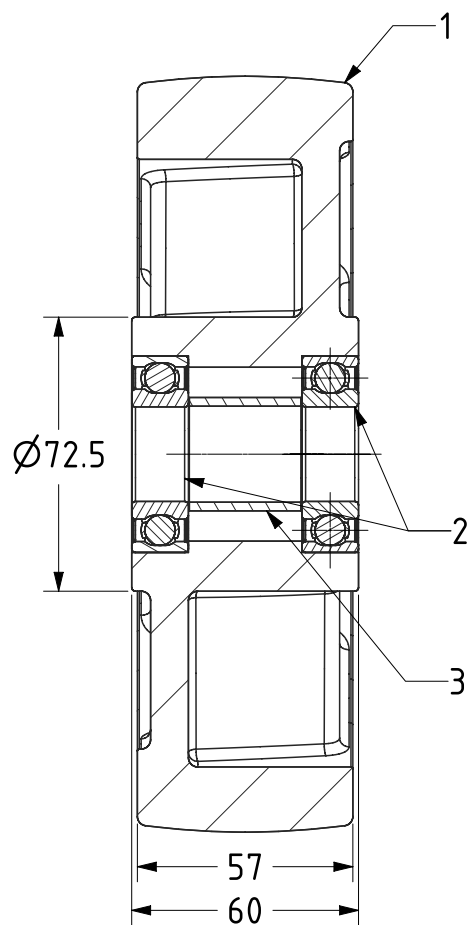
SECTION A-A
