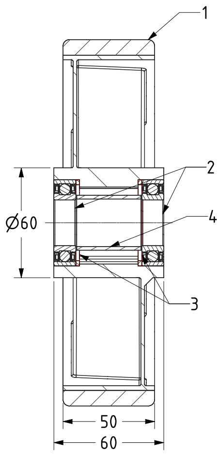
SECTION A-A
