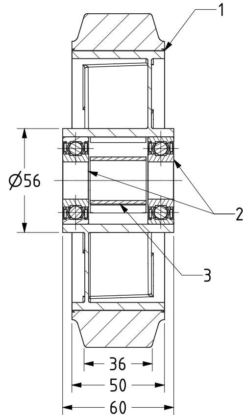
SECTION A-A
