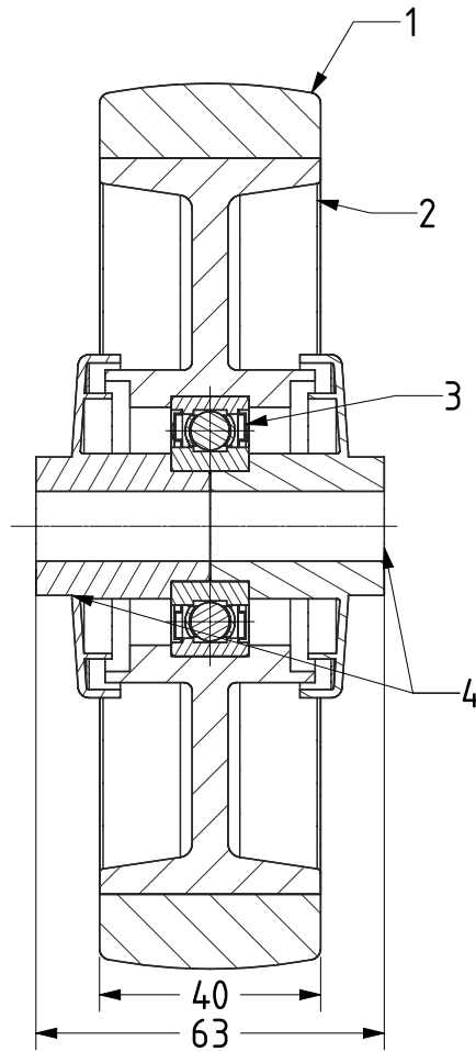
SECTION A-A
