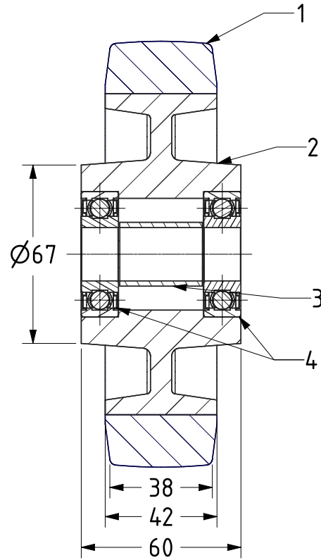
SECTION A-A
