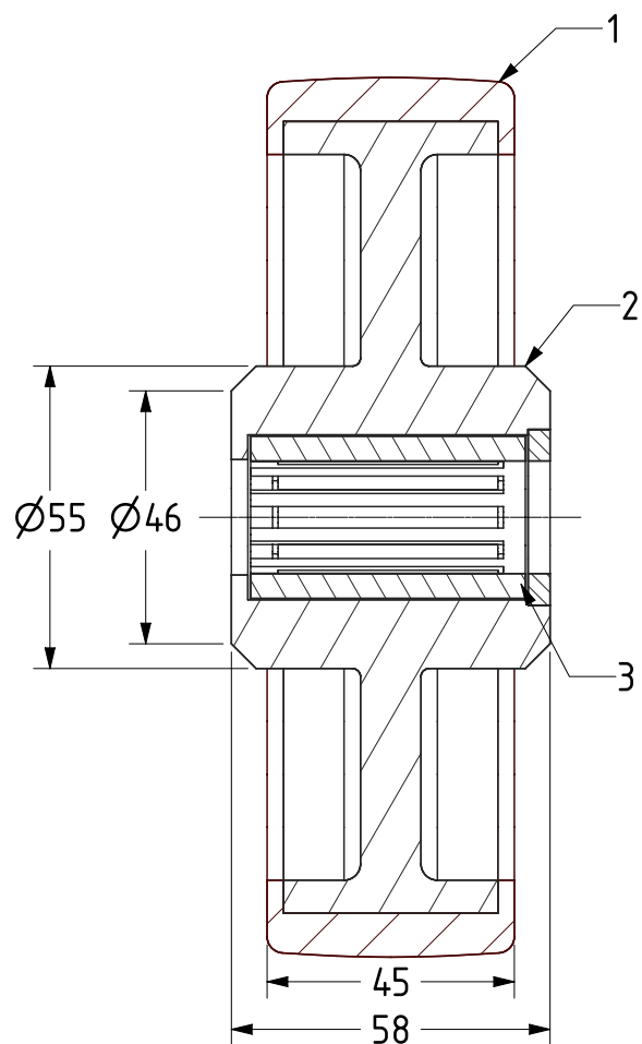
SECTION A-A
