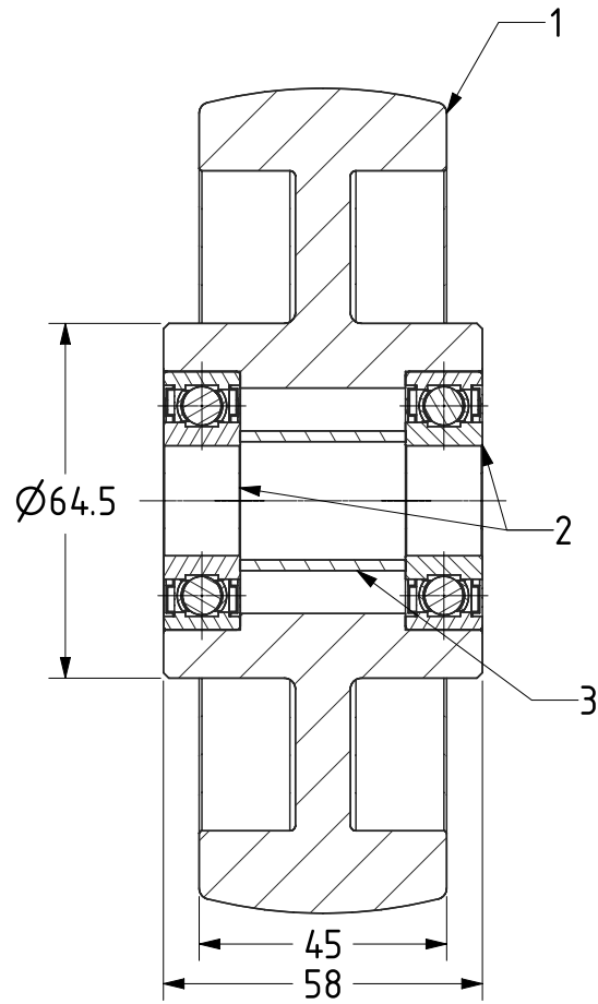
SECTION A-A
