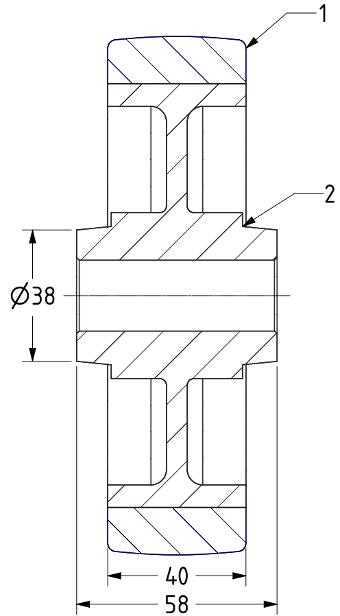
SECTION A-A
