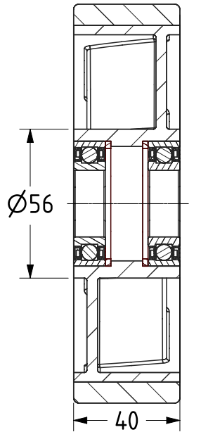
SECTION A-A
