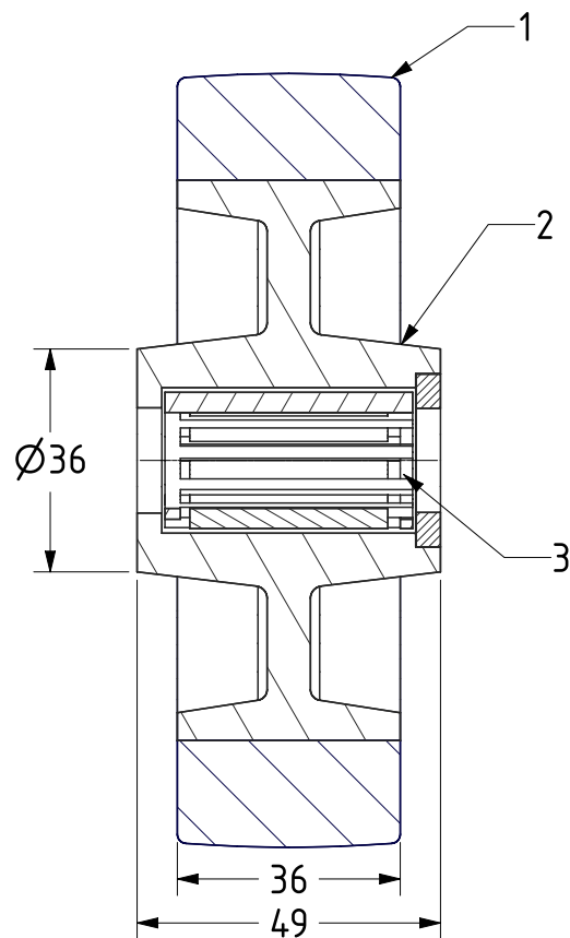
SECTION A-A
