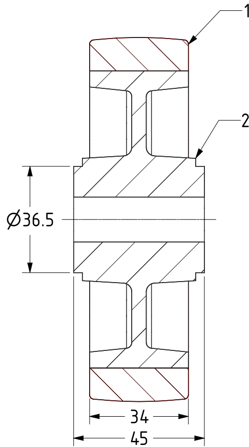
SECTION A-A
