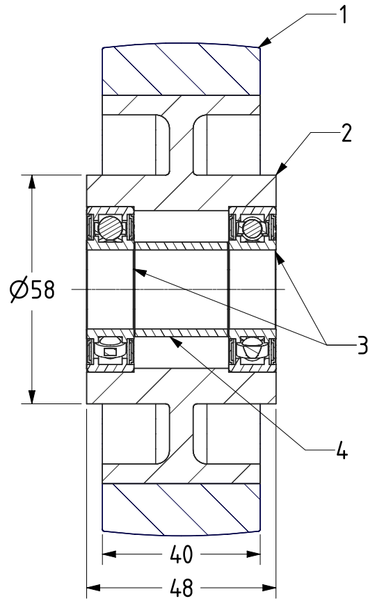
SECTION A-A
