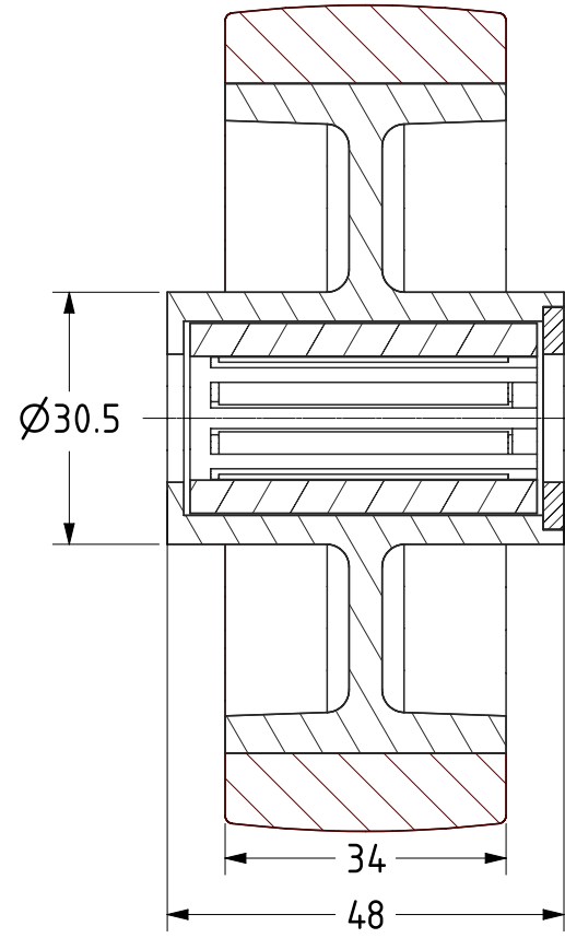
SECTION A-A
