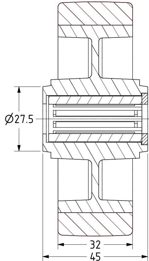
SECTION A-A
