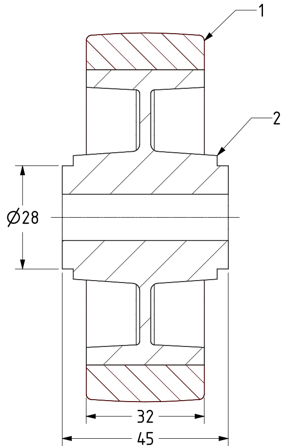
SECTION A-A
