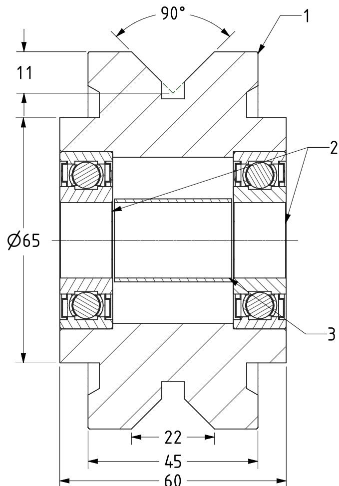
SECTION A-A
