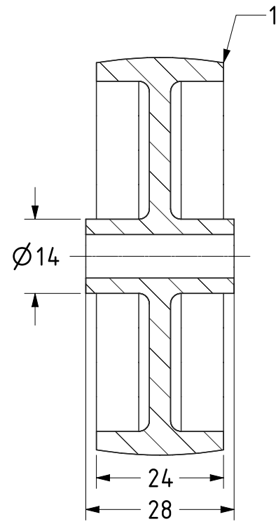
SECTION A-A
