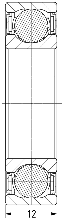
SECTION A-A
