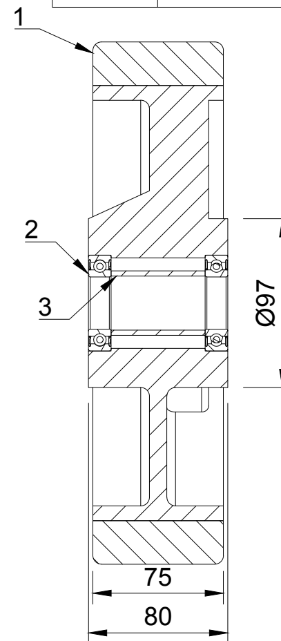
A-A (1:3)
