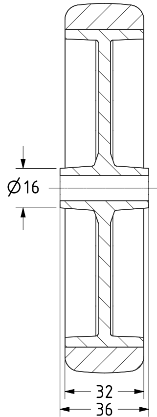
SECTION A-A
